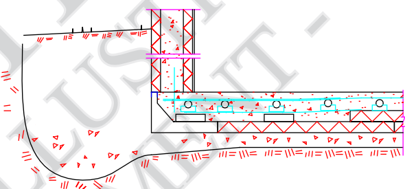
Mur de CIB partiellement enterré
