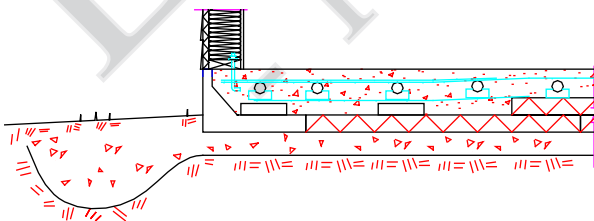
Mur encadrer de bois fini en revêtement
