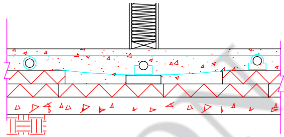
Section de dalle - Mur porteur
