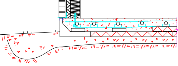
Mur encadrer de bois fini en briques
