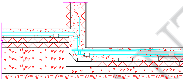
Section de dalle marchée
