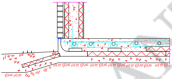
Mur de CIB fini en briques - Dalle avec bordure isolante
