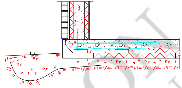
Mur de CIB fini en briques
