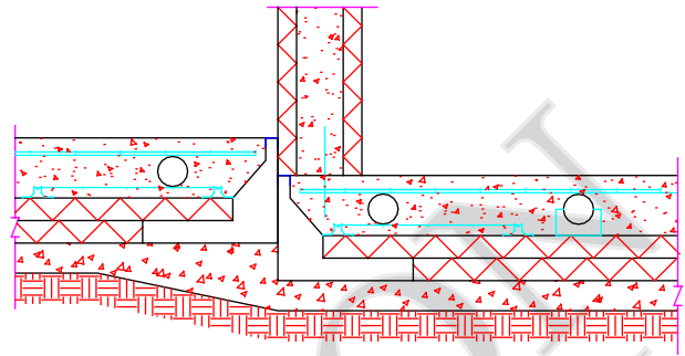
Pas entre dalles chauffées
