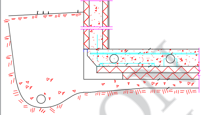
Mur de CIB partiellement enterré
