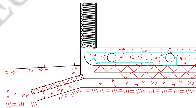
Mur encadrer de bois fini en revêtement - Dalle avec bordure isolante
