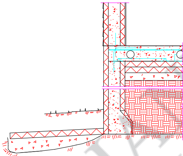
Dalle chauffée élevée - Dalle avec bordure isolante
