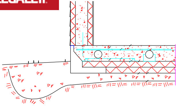
Mur de CIB fini en revêtement
