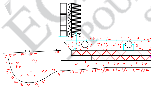
Mur encadrer de bois fini en briques
