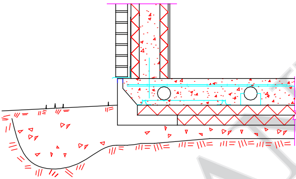
Mur de CIB fini en briques
