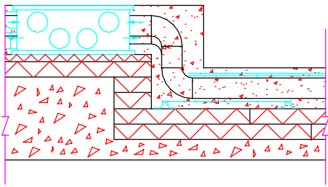
Section de dalle marchée
