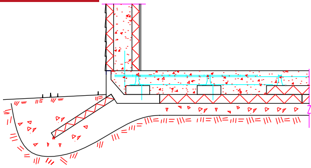
Mur de CIB fini en revêtement Bâtiment chauffée sur dalle de 5" non chauffée avec bordure isolante
