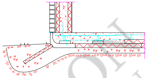
Mur de CIB fini en briques Bâtiment chauffée sur dalle de 5" non chauffée avec bordure isolante
