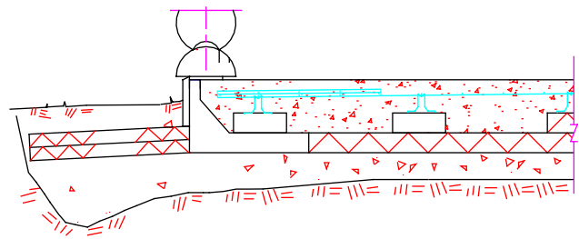
Mur de bûches avec bûche de base 1/2 complet Bâtiment chauffée sur dalle de 5" non chauffée avec bordure isolante
