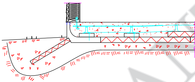
Mur encadrer de bois fini en revêtement Bâtiment chauffée sur dalle de 5" non chauffée avec bordure isolante
