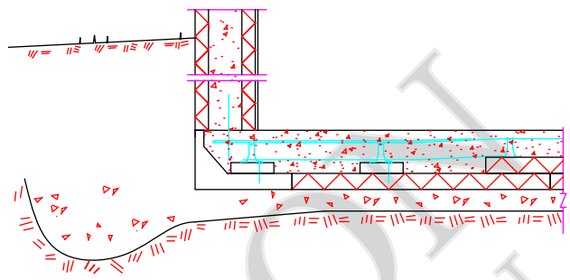
Bâtiment non chauffée sur dalle de 5" enterré non chauffée
