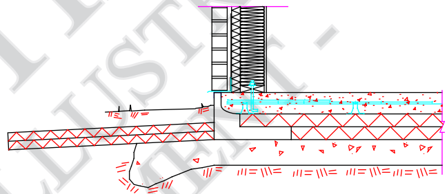
Mur encadrer de bois fini en briques Bâtiment non chauffée sur dalle de 5" non chauffée avec bordure isolante
