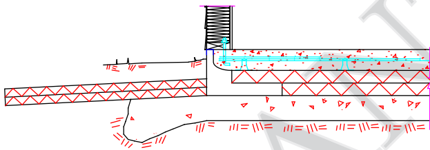
Mur encadrer de bois fini en revêtement Bâtiment non chauffée sur dalle de 5" non chauffée avec bordure isolante
